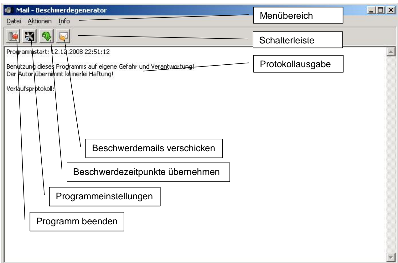
Abbildung 1: Programm-Oberfläche
