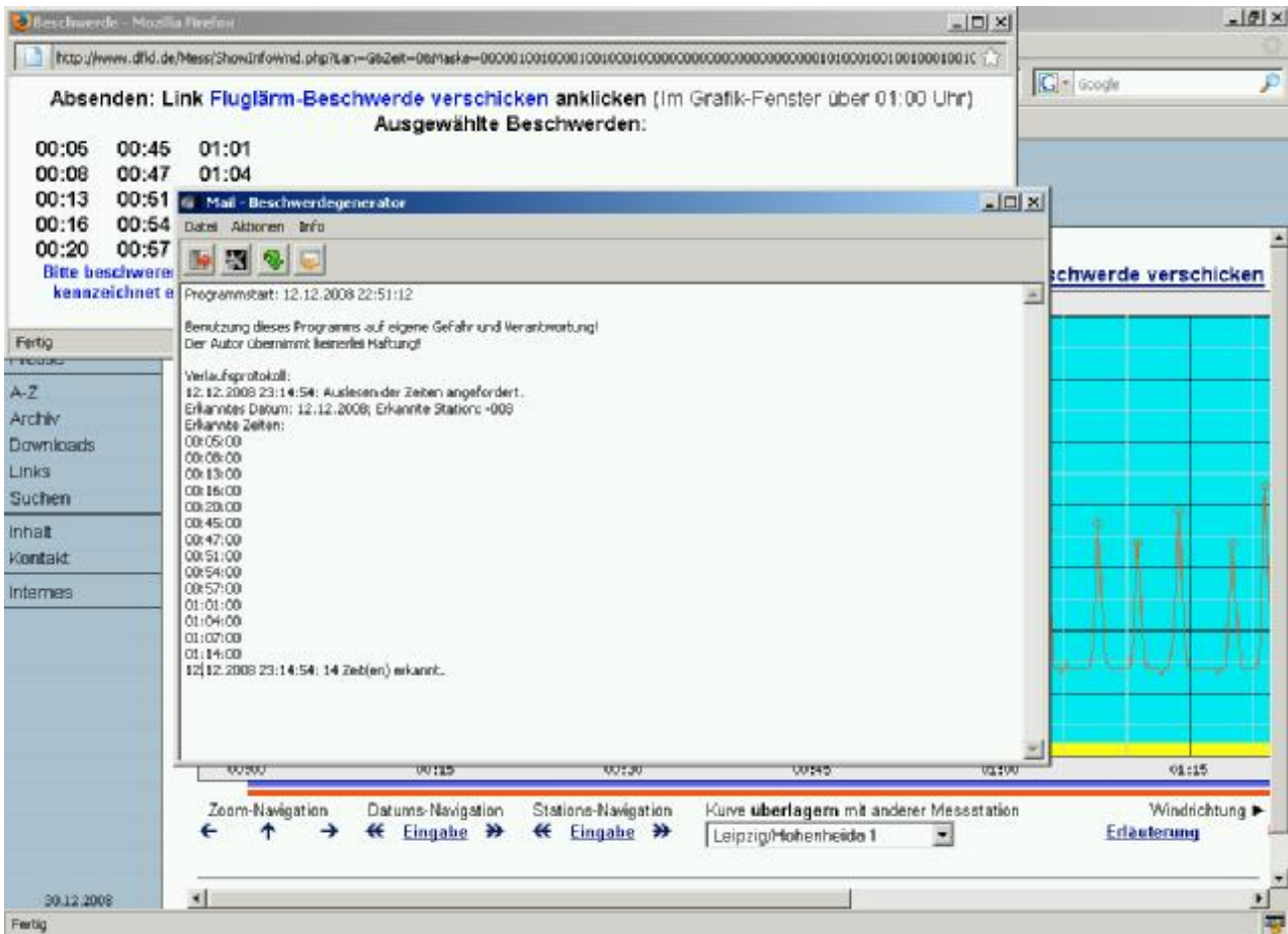
Abbildung 6: Ausgelesene Beschwerdezeitpunkte
