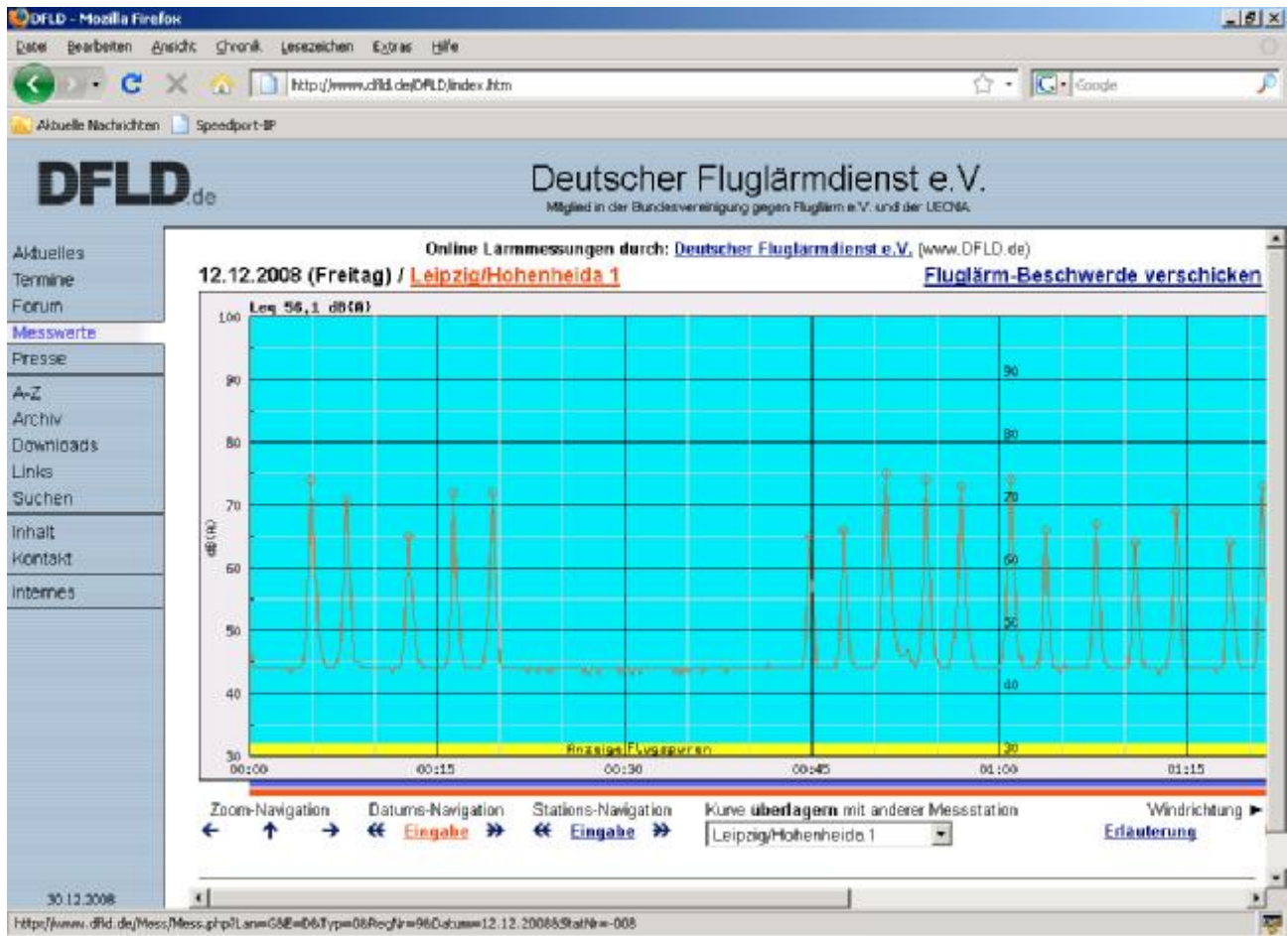
Abbildung 4: Zoombereichsansicht
